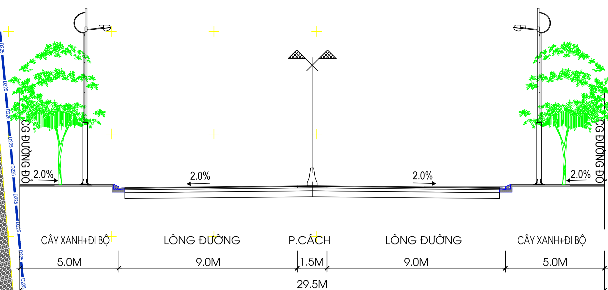
MẶT CẮT A-A (QUỐC LỘ 1A)
