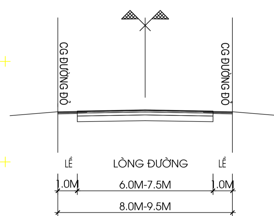
MẶT CẮT 2-2
