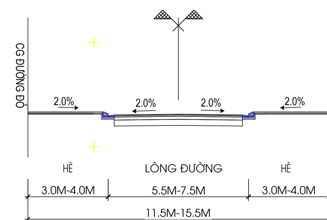
MẶT CẮT 1-1
